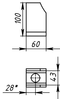
Поз.4 (Ушко)
