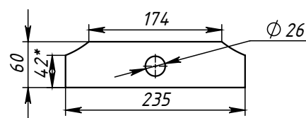
Поз.4 (Ушко) развертка
