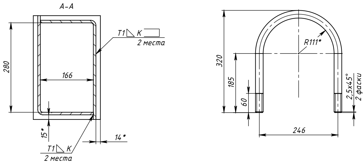
Поз.5 (Хомут)
