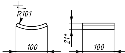
Поз.6 (Упор)
