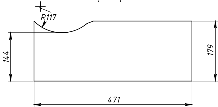
Поз.2 (Угольник) развертка
