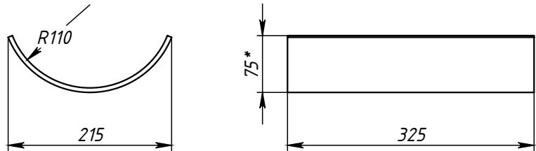
Поз.3 (Ложемент)
